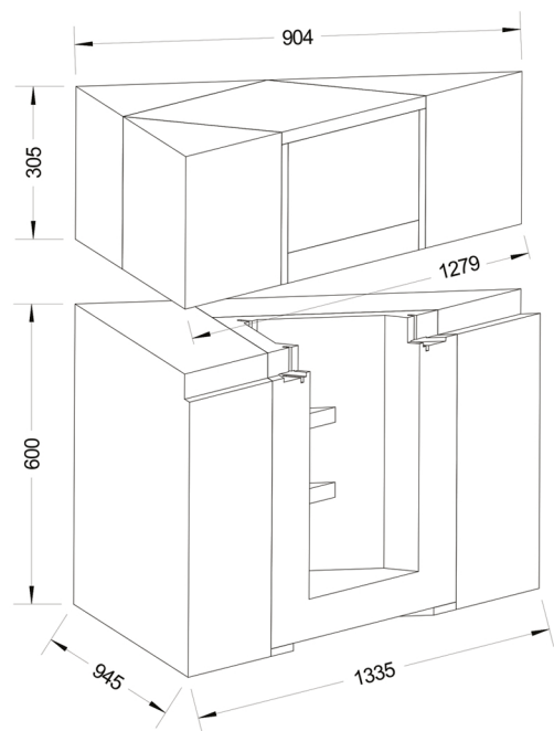
Eckmodul für Wannengröße 180 x 85 cm
