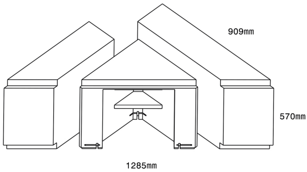
Eckfüllstück für Wannengröße 170 x 75 cm
