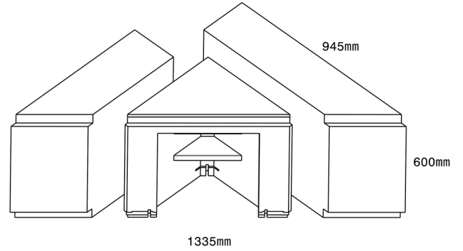
Eckfüllstück für Wannengröße 180 x 85 cm
