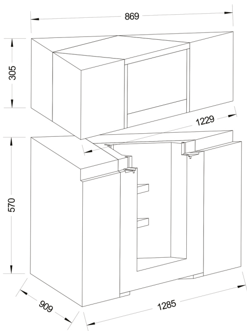
Eckmodul für Wannengröße 170 x 75 cm
